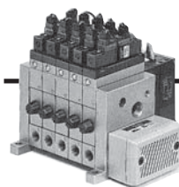
ZZM 真空组件位数 - S 消声器位置
