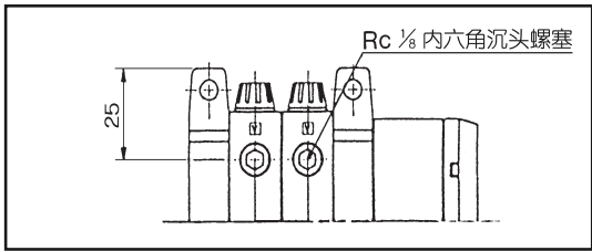
VAC□引出位置:侧面引出的场合(下面真空口带螺塞)
