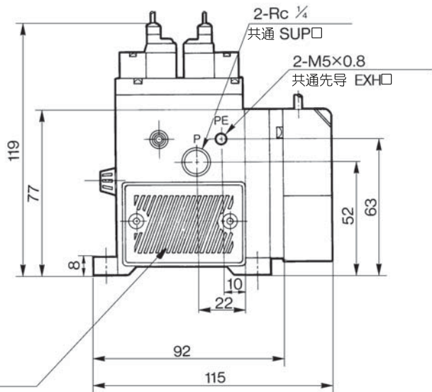
集成式专用消声器 (ZZM-SA)
