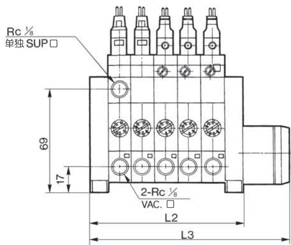
集成式专用消声器 (ZZM-SA)
