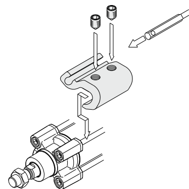
• D-A9□(V)、M9□(V)、M9□W(V)、 M9□A(V)型的安装示例。
