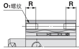
两端螺孔式: CQ2A・CDQ2A
