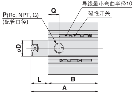
无杆侧带凸台
