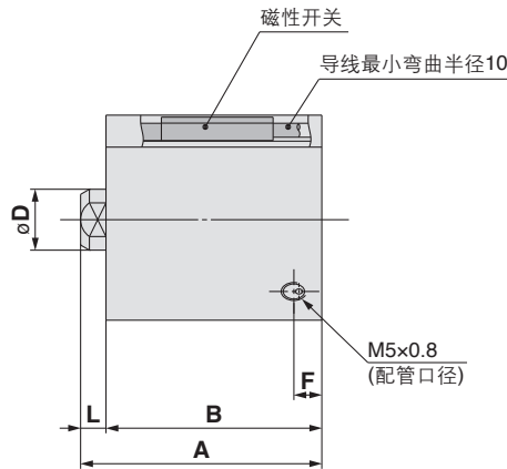
无杆侧带凸台
