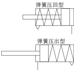
JIS图形符号
