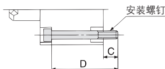
弹簧压出型
