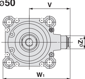
内置快换接头型/ ø32~ø50
