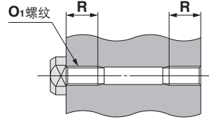
两端螺孔式: CDQ2A
