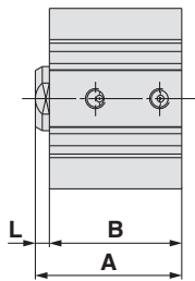
单杆 · 双作用
