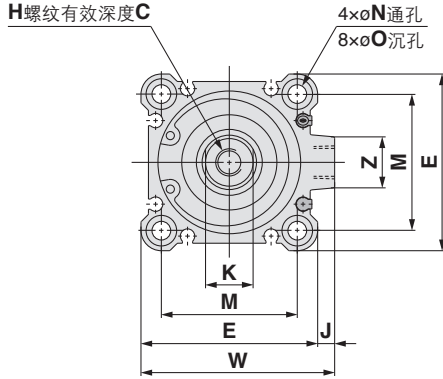
标准型(通孔式)/ CQ2B・CDQ2B
